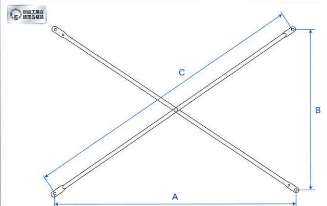
筋違 組合せ表
